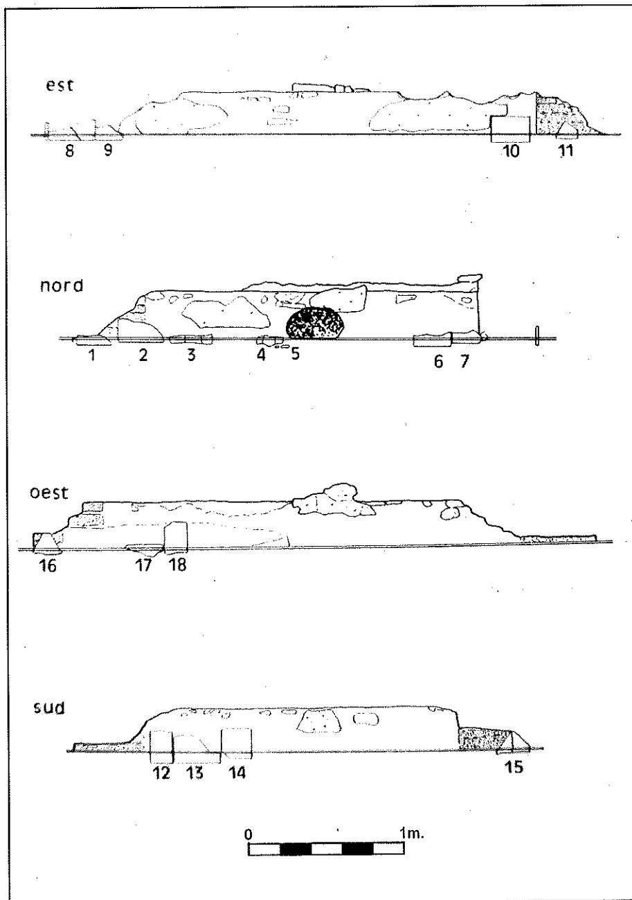
16.- Alçats dels paraments exteriors de l'impluvi de Torre Llauder, amb indicació numerada de les crustae reaprofitades (dibuix J.F. Clariana).
