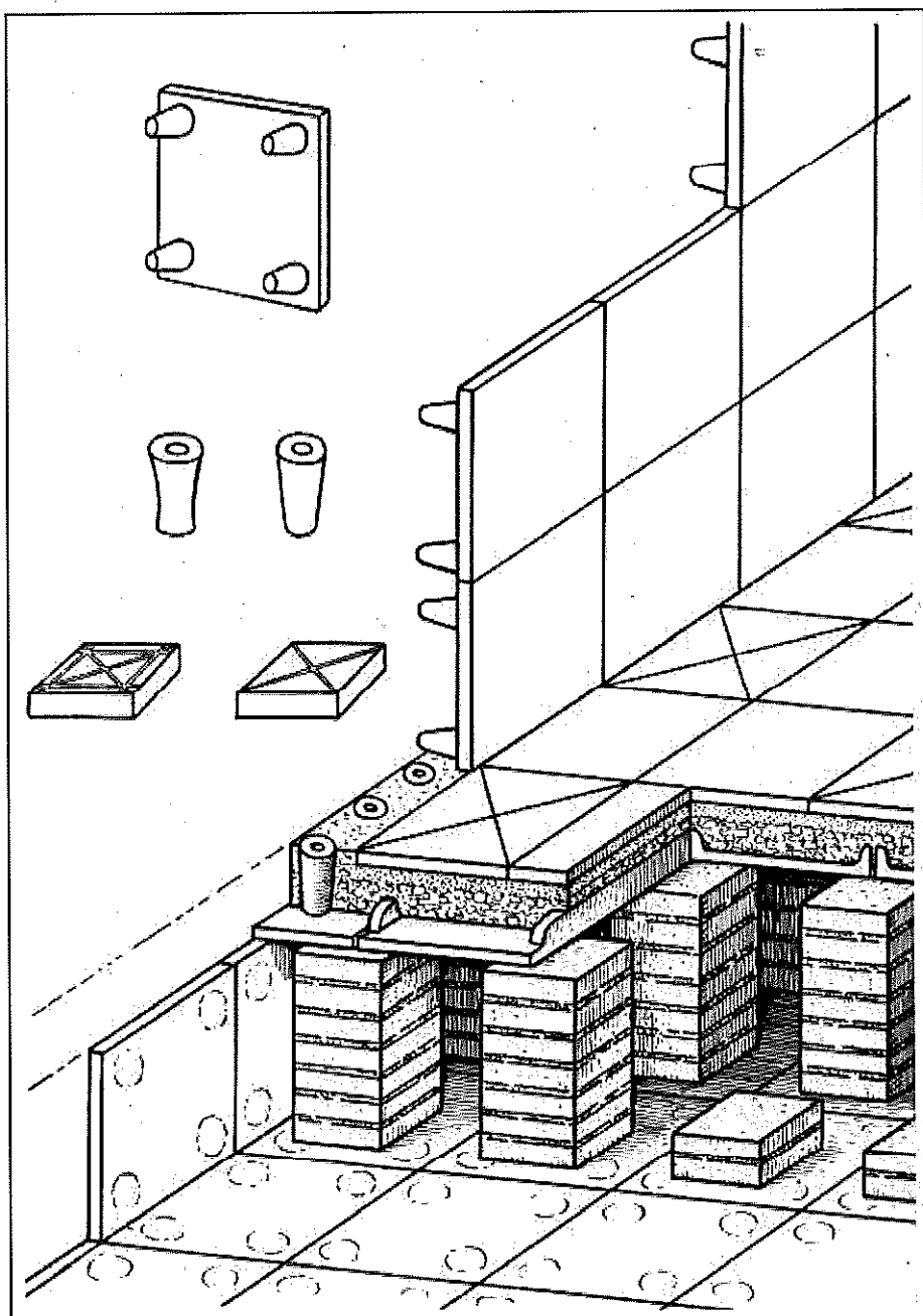
5.- Reconstrucció ideal del sistema constructiu de l'hipocaust (dibuix M. Ribas).
