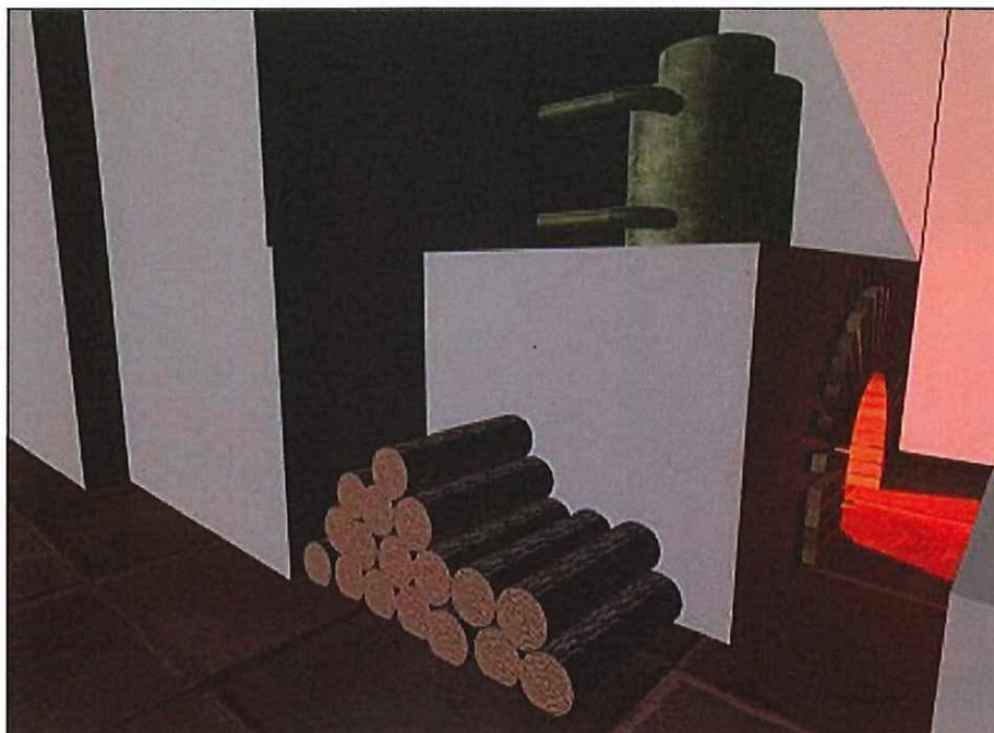
17.- Reconstrucció 3D del sistema de caldera de l'hipocaust 1 de Torre Llauder (dibuix F. Bayés).
