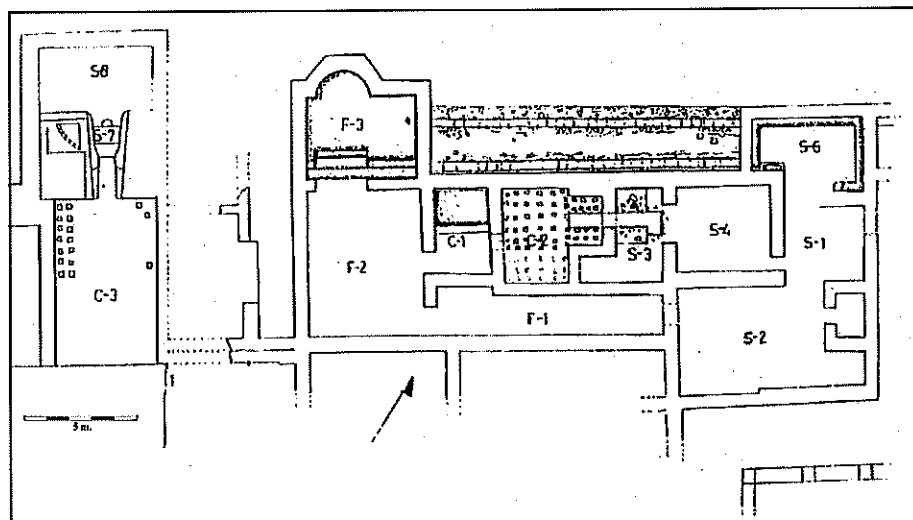
2.- Planta dels balnea de Torre Llauder (dibuix Ll. Piñol 1993)
