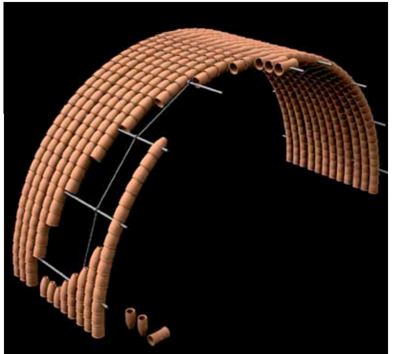
Recreació 3D del sistema constructiu de la coberta del caldarium amb tubs afusats
