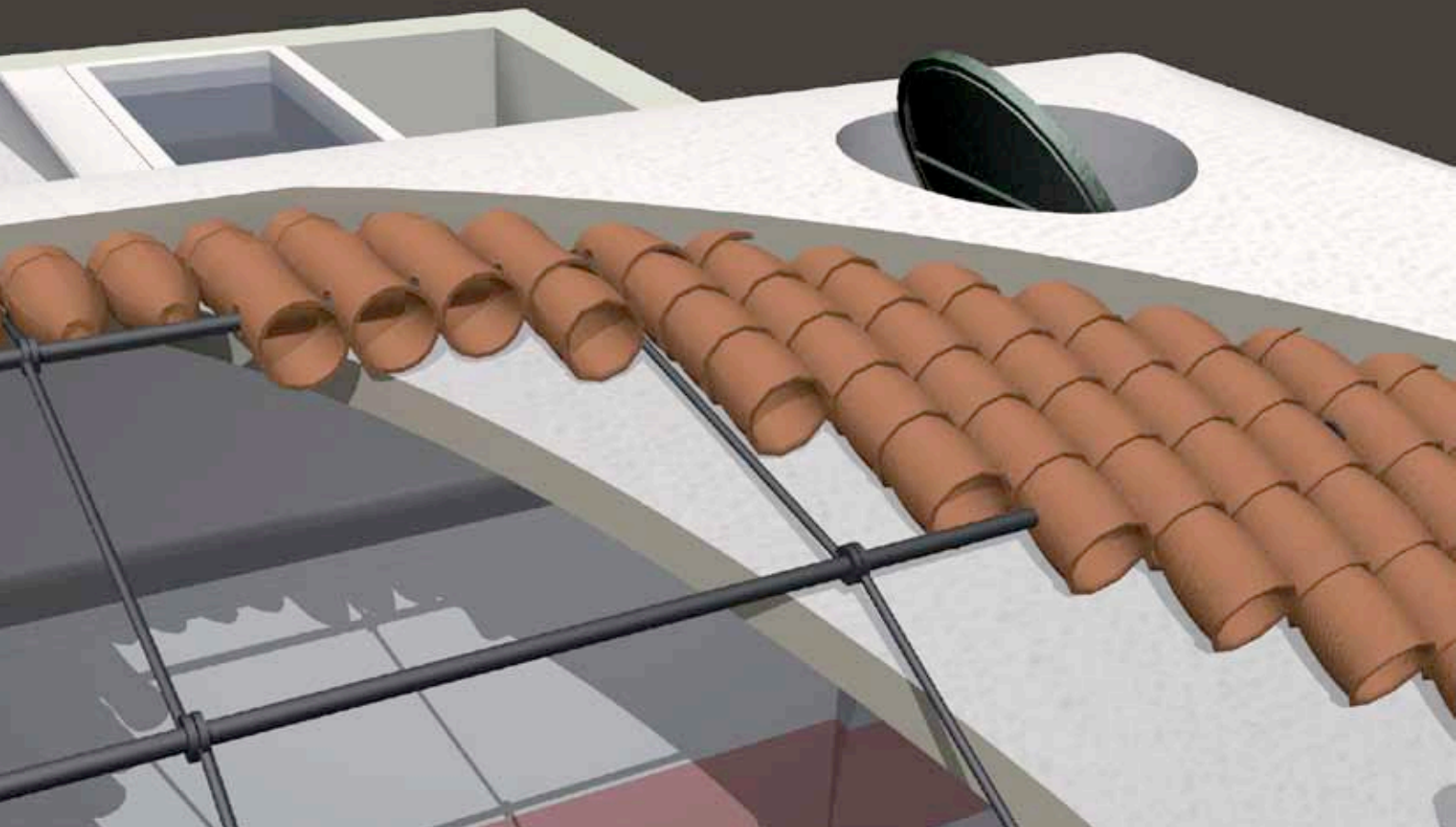
Detall constructiu de la coberta del caldarium
