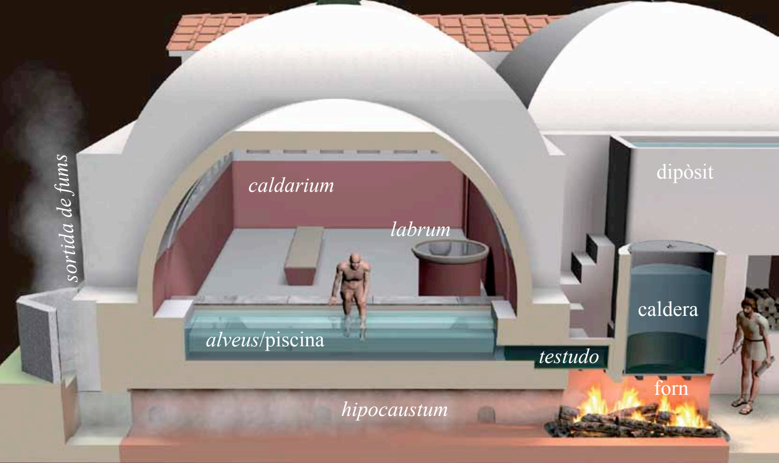
Secció hipocaustum, alveus, testudo, caldera i forn dels banys d'Ilturo
