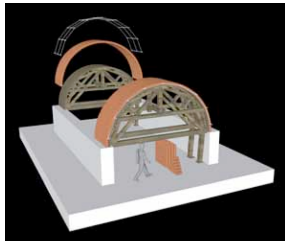
Detall constructiu de la coberta del caldarium amb bastides o cintres mòbils
