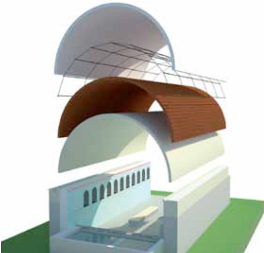
Sistema constructiu de la coberta del caldarium
